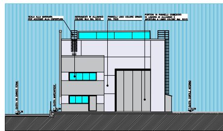
PROSPETTO NORD
